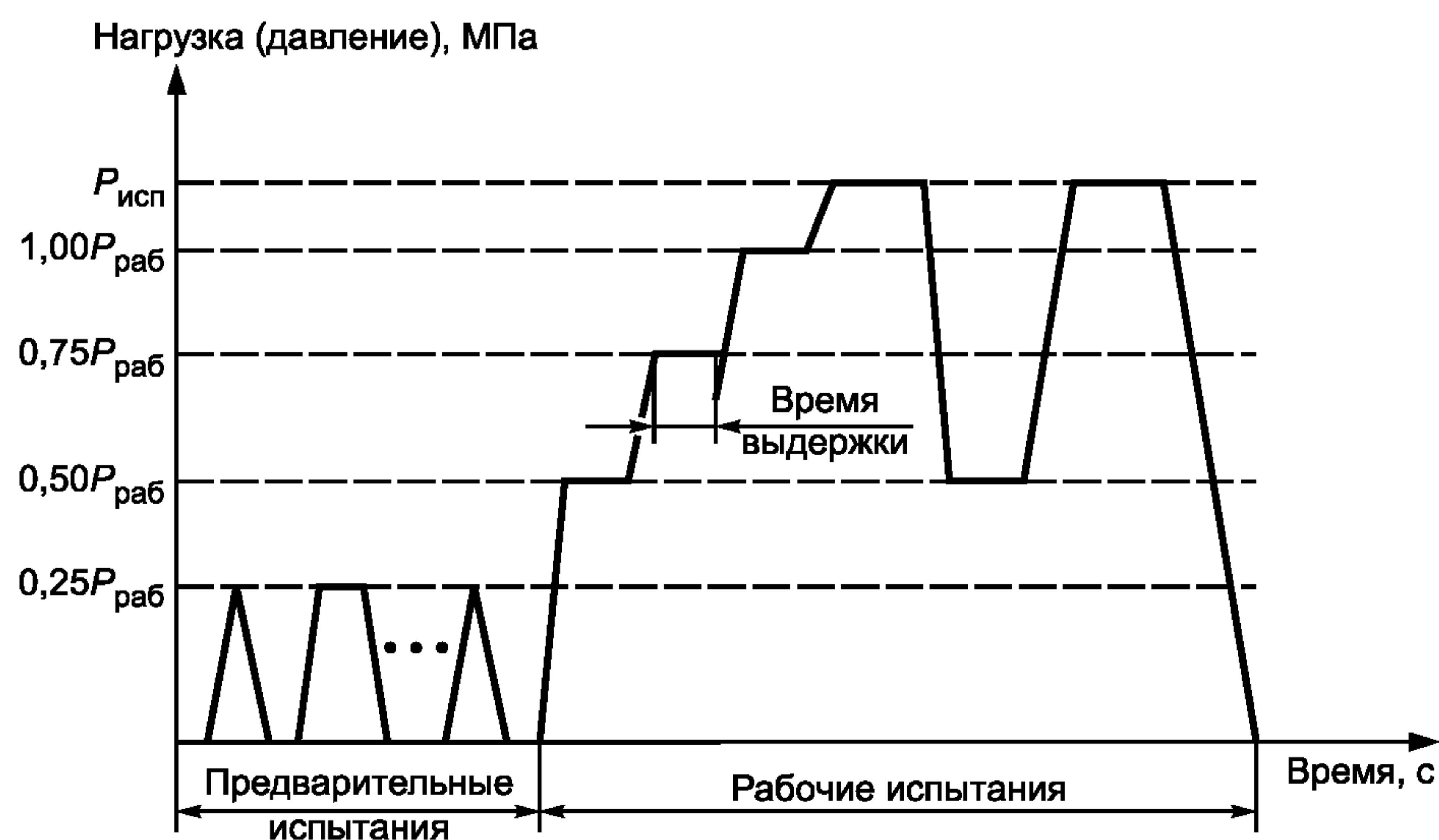
Рисунок 1 — Типовой график нагружения
